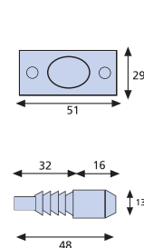
Hinge Bolt
